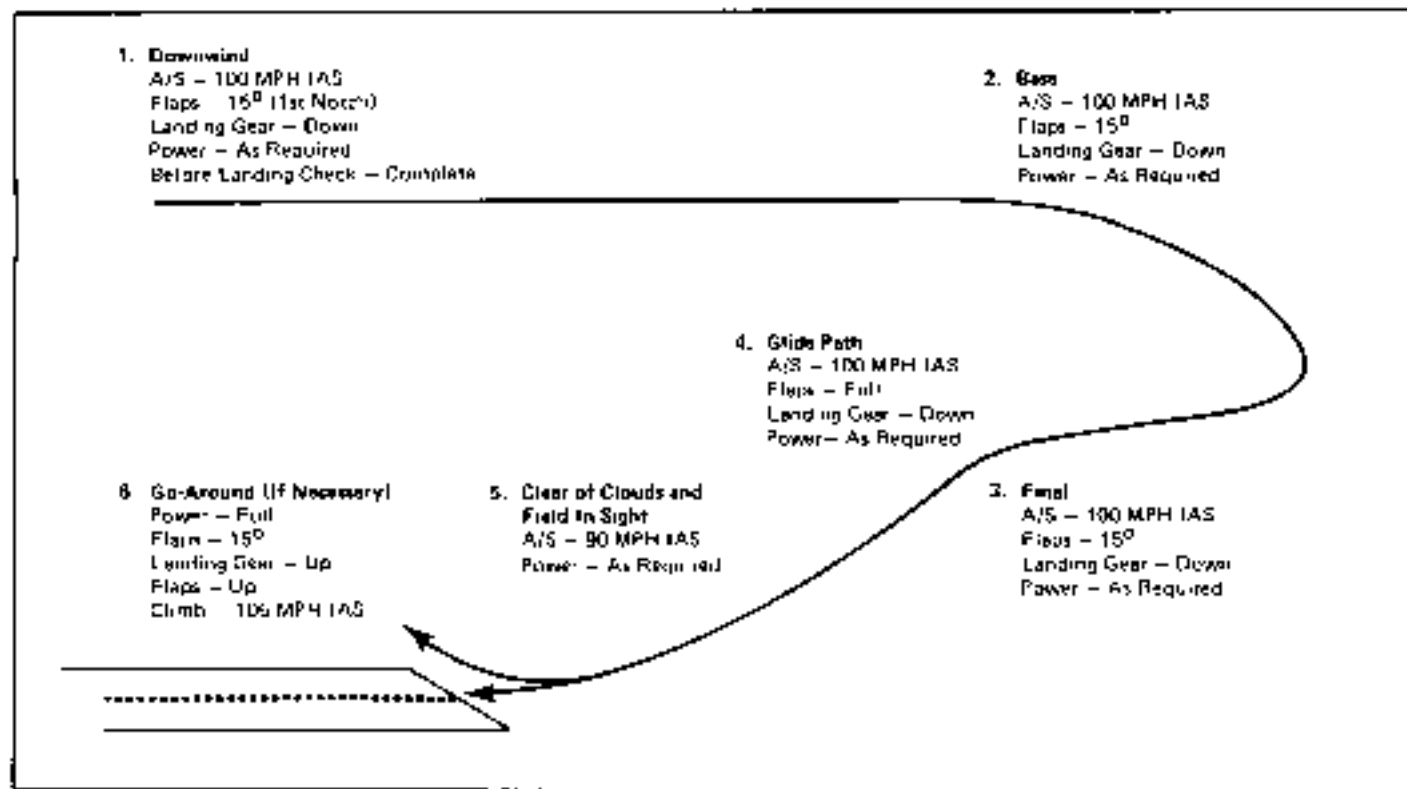
Figure 8-2 PAR Approach
